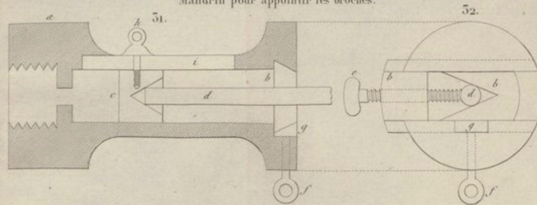
Mandrin pour appointir les broches.
