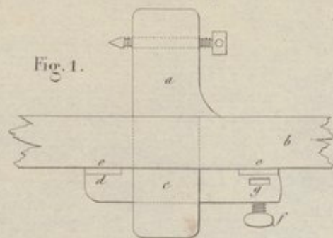
Coins à vis de répulsion.
