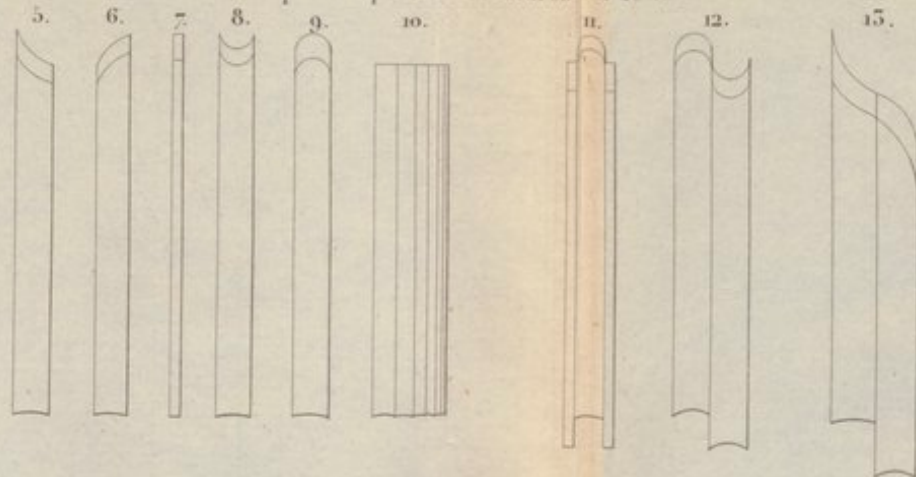
Compositeur pour les moulures sur le tour.
