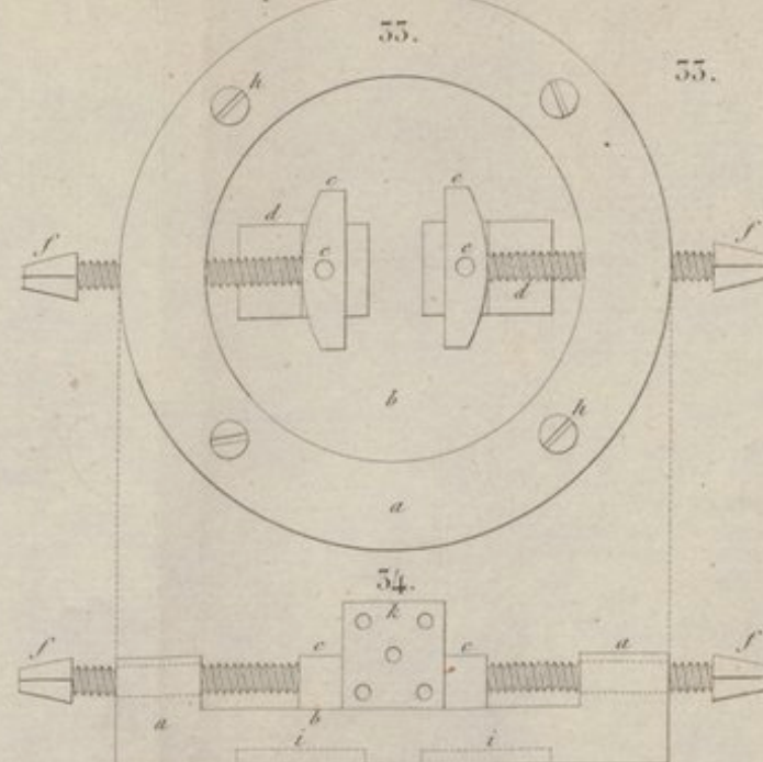
Mandrin pour tourner les cubes.
