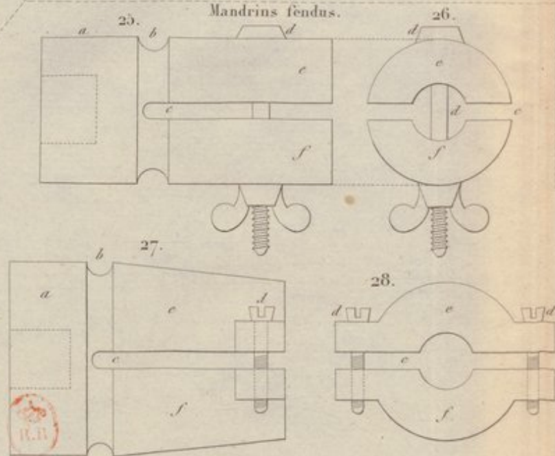
Mandrins fendus.
