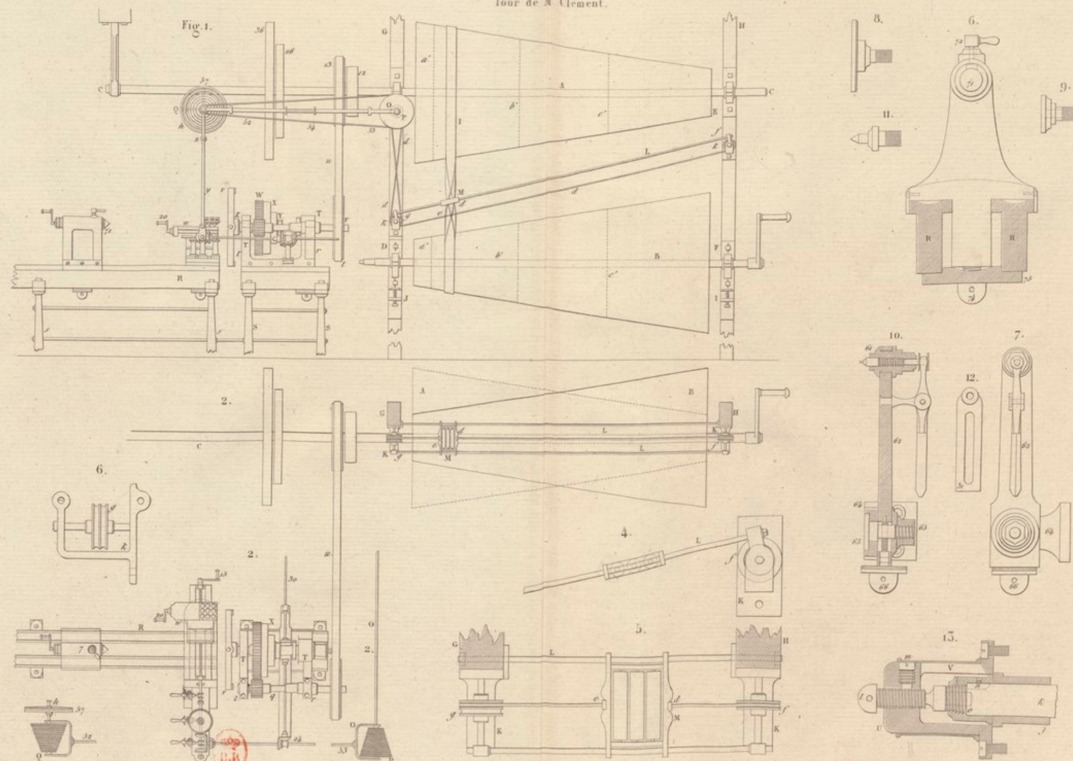
Tour de M. Clément.
